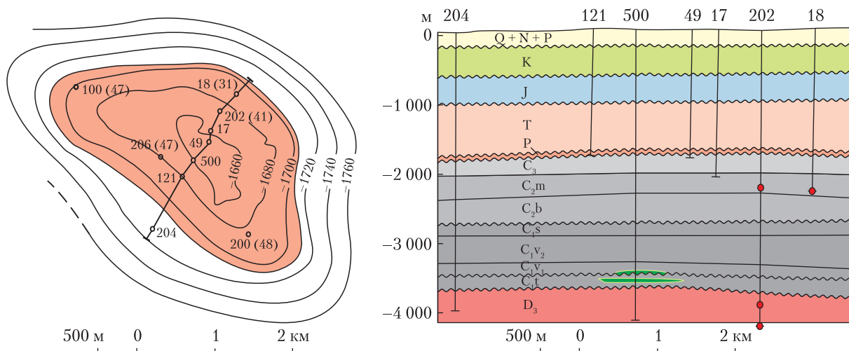
Рис. 2. Леляківське родовище. Схема глибин залягання продуктивного горизонту та розташування свердловин, у яких розраховані значення теплового потоку (в дужках). Геологічний розріз, розміщення свердловин та точки, в яких виконано заміри [4]
