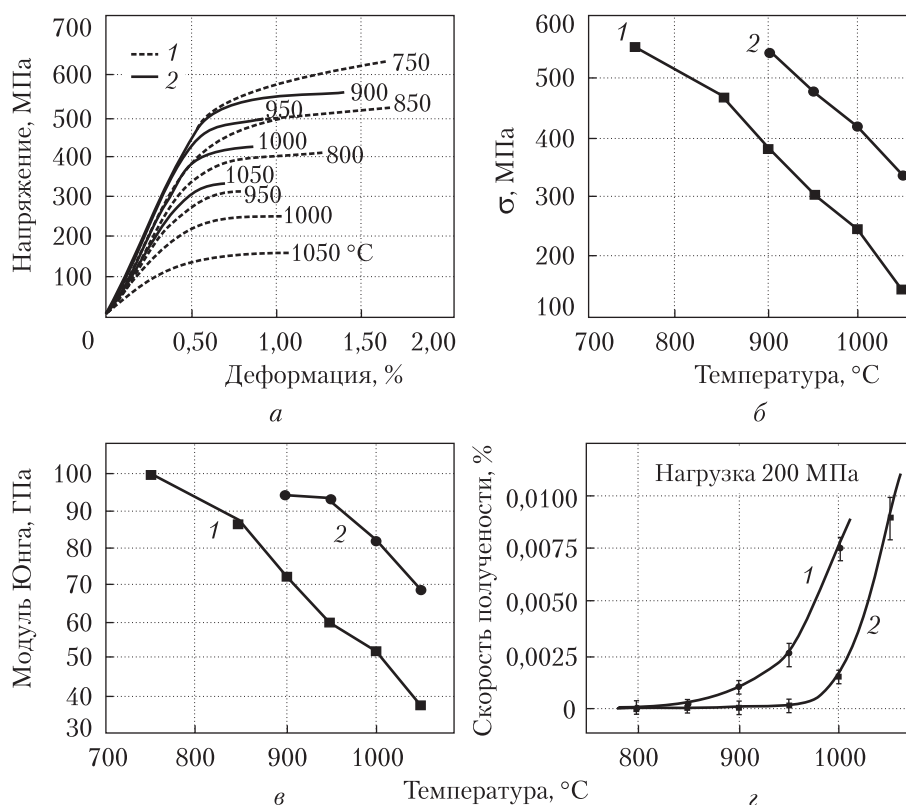
Рис. 4. Зависимость физико-механических свойств литых (1) и после БЗП (2) сплавов от температуры: а – кривые деформации; б – предел текучести; в – модуль Юнга; з – ползучесть
