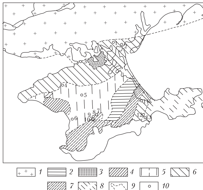
Рис. 1. Схематична мапа докрейдової поверхні Рівнинного Криму та Присивашшя (за [2], із доповненням автора): 1 – докембрійські утворення; 2 – палеозой-верхньопротерозойські; 3 – пермо-тріасові; 4 – верхньотріасові – нижньоюрські; 5 – нижньо- і середньоюрські (?); 6 – середньоюрські; 7 – середньо- і верхньоюрські (?); 8 – верхньоюрські; 9 – ймовірні межі стратиграфічних комплексів; 10 – свердловини. Цифрами на мапі позначені свердловини: 1 – Новоолексіївська Р-1; 2 – Генічеська-5; 3 – Красноперекопська-2; 4 – Березівська-4; 5 – Новоселівська Р-1; 6 – Миколаївська-1; 7 – Зуйська-9; 8 – Зуйська-26; 9 – Зуйська-30; 10 – Зуйська-33; 11 – Шубинська-7; 12 – Журавкинська-1; 13 – Південно-Видненська-1
