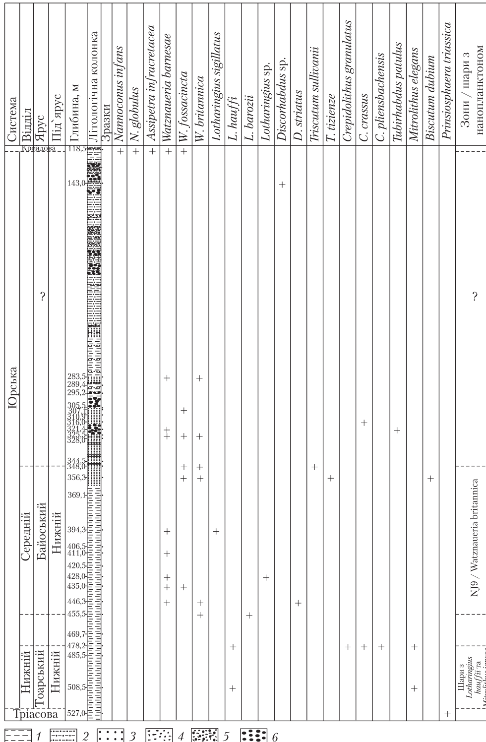
Рис. 2. Стратиграфічне поширення вапнякового нанопланктону у відкладах свердловини Зуйська-30. Умовні позначення: 1 – аргіліти; 2 – алевроліти; 3 – пісковики; 4 – гравеліти; 5 – гравеліти піщаністі; 6 – конгломерати
