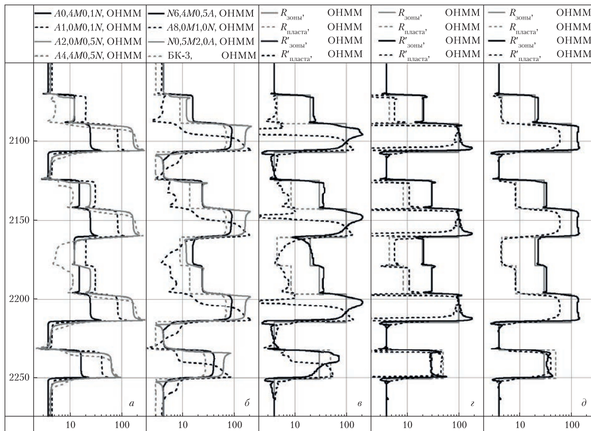
Рис. 3. Скважина “Тестовая-1” (УС бурового раствора 1 Ом · м). а, б – диаграммы УО зондов комплекса; в – результат обратной задачи, если все K=1 ; г – K_{A4,0M0,5N}=0 , K_{A8,0M1,0N}=0 ; д – K_{A4,0M0,5N}=0 , K_{A8,0M1,0N}=0 но K_{7F1,6}=1
