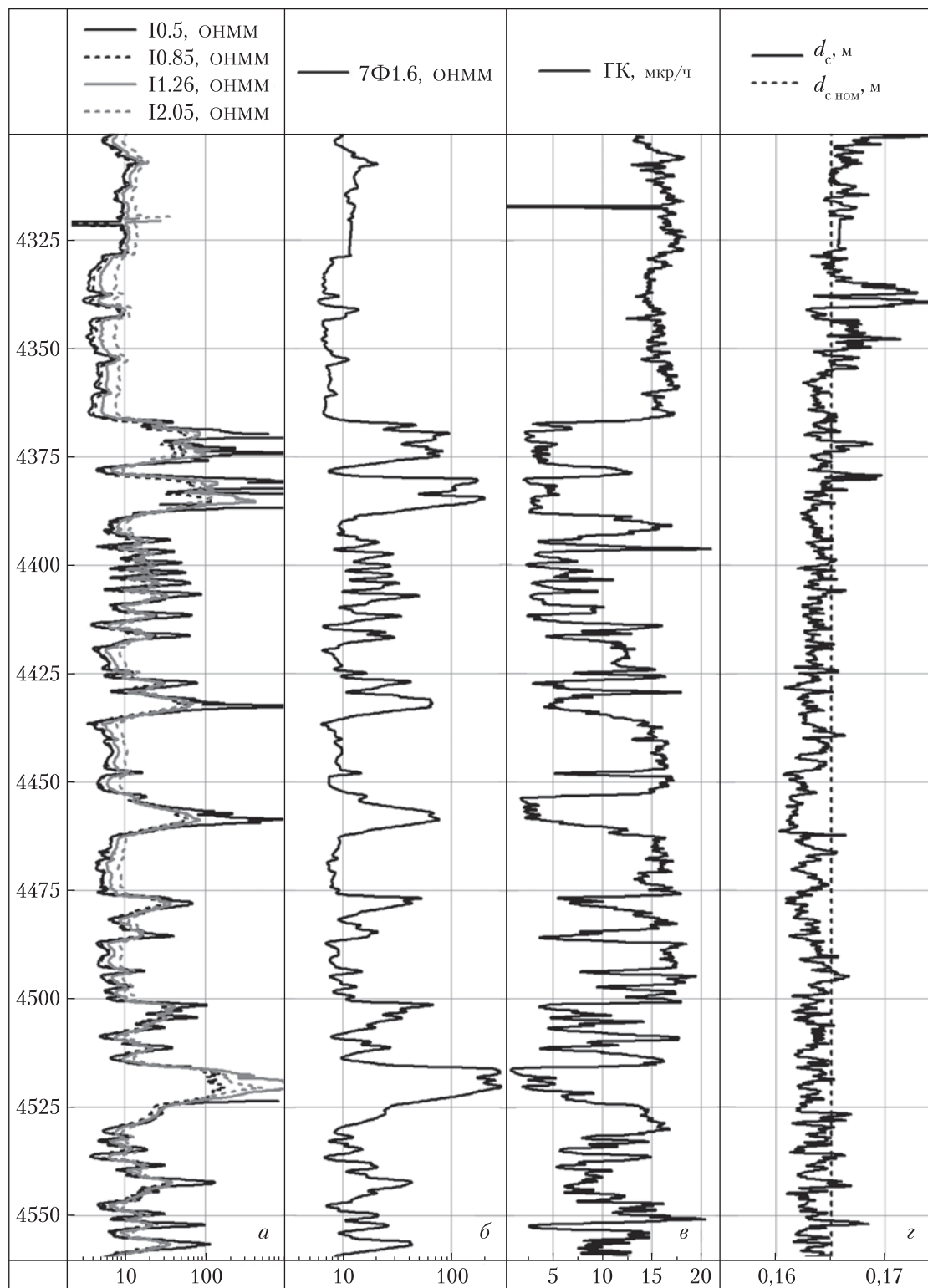
Рис. 2. Скв. Островерховская-28. Каротажные диаграммы: а – 4ИК; б – 7Ф1.6; в – ГК; z – карвернометрия
