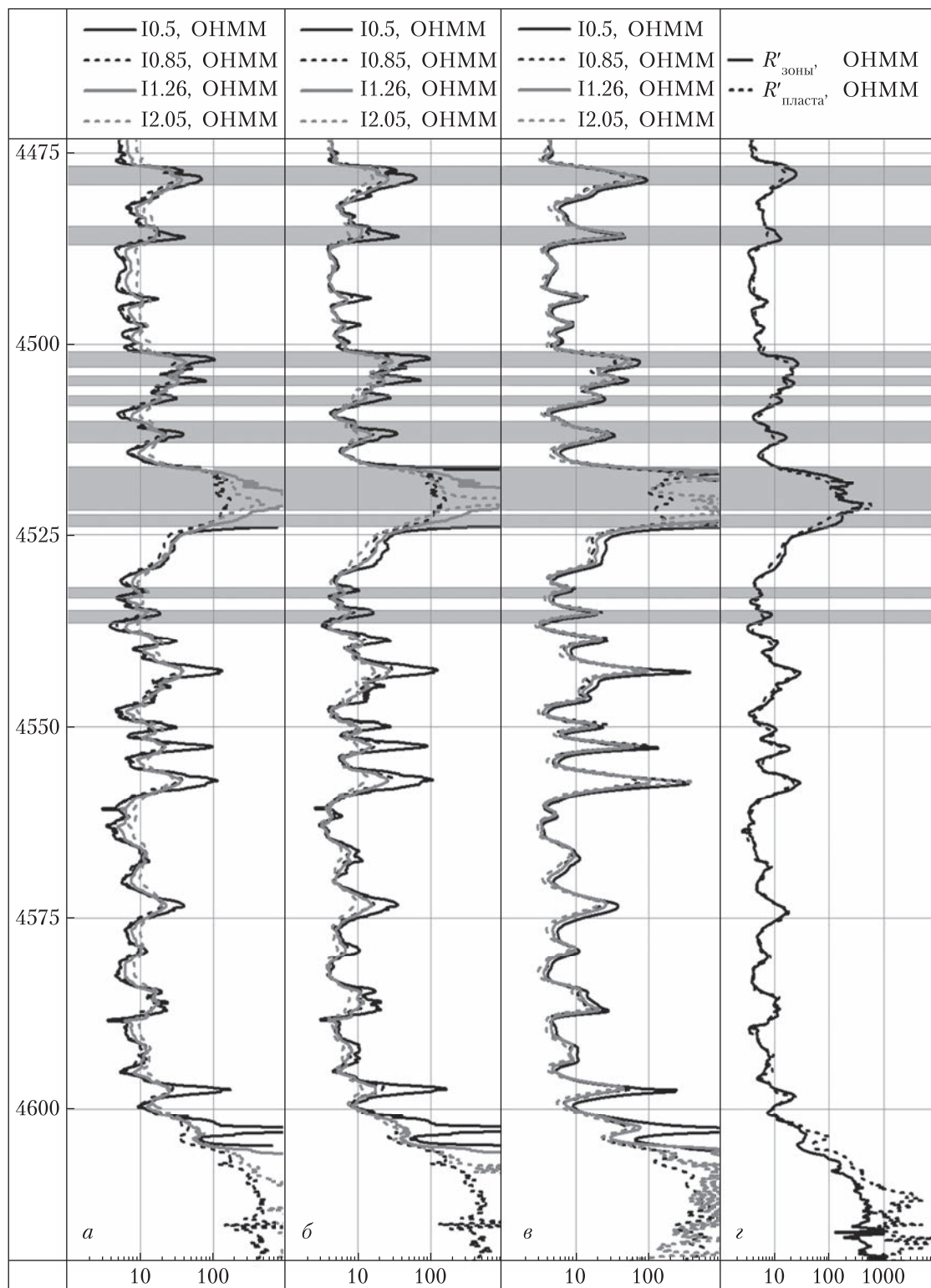
Рис. 3. Скв. Острореховская-28: a – измеренные КС; б – УС после внесения поправки “за скин-эффект”; в – УС после учета влияния вмещающих пластов; г – результат решения обратной задачи
