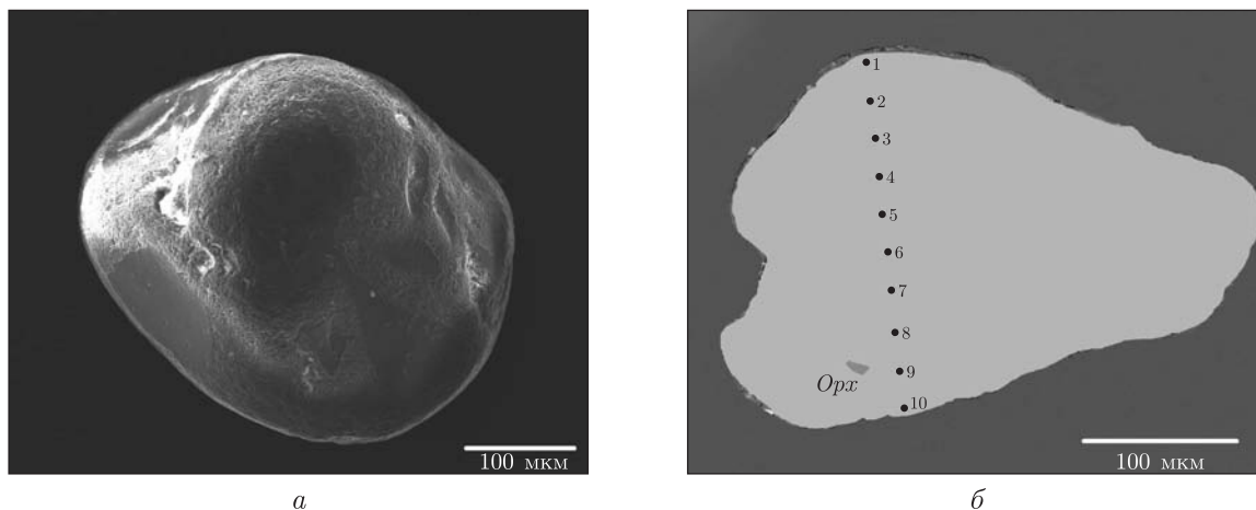
Рис. 1. Зональний піроп із руслового алювію середньої течії р. Уборть (РЕМ-знімки): а — загальний вигляд; б — полірований зріз (точки аналізу 1–10 на мікрофотографії відповідають номерам аналізів у табл. 1; Orx — включення ортопіроксену)
